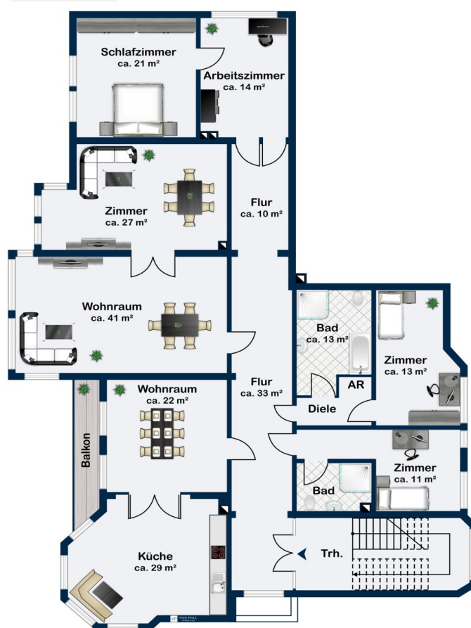
2. Obergeschoss
