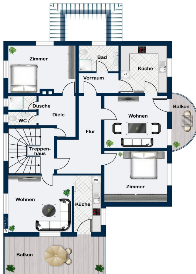
Obergeschoss
