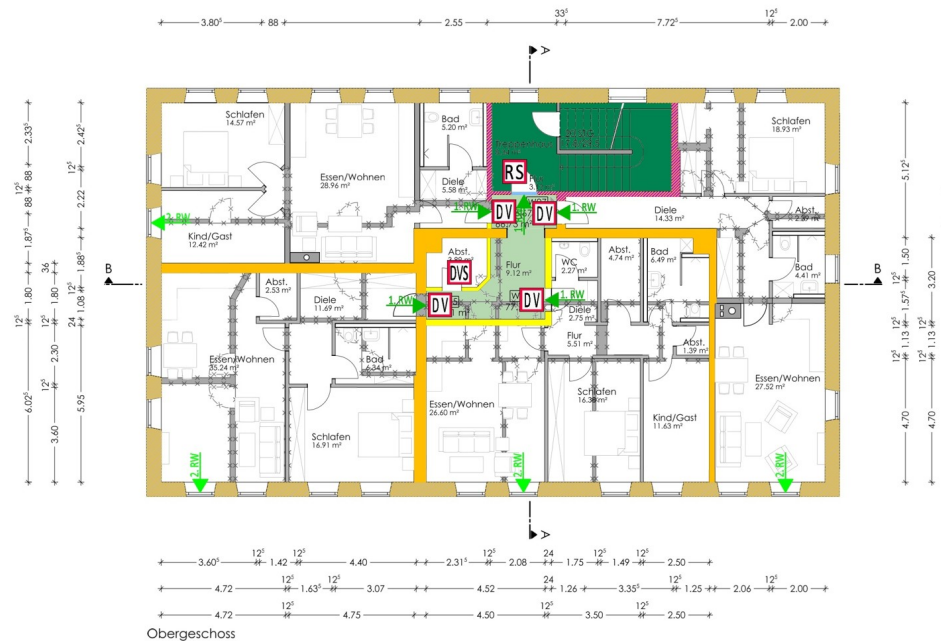
Obergeschoss
