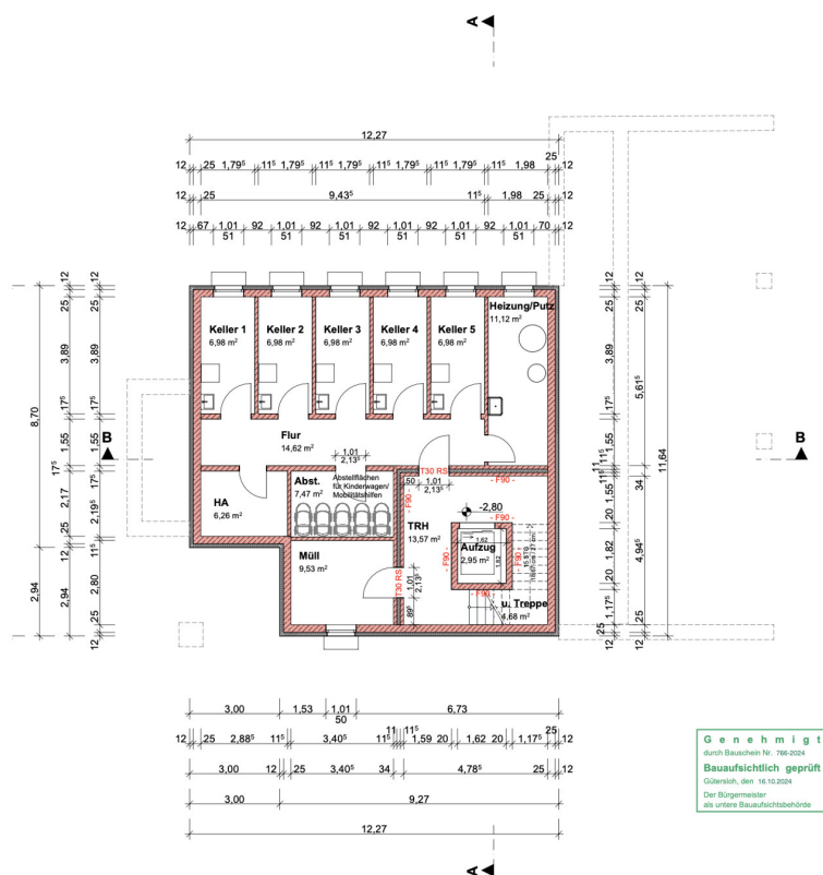
GRUNDRISS UG
