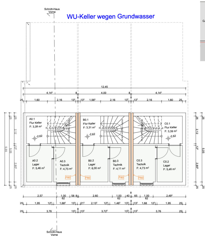
UG-vorderes Haus M 1.100
