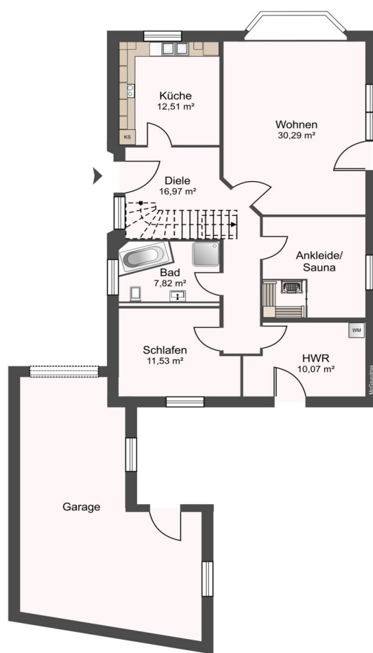
Erdgeschoss
