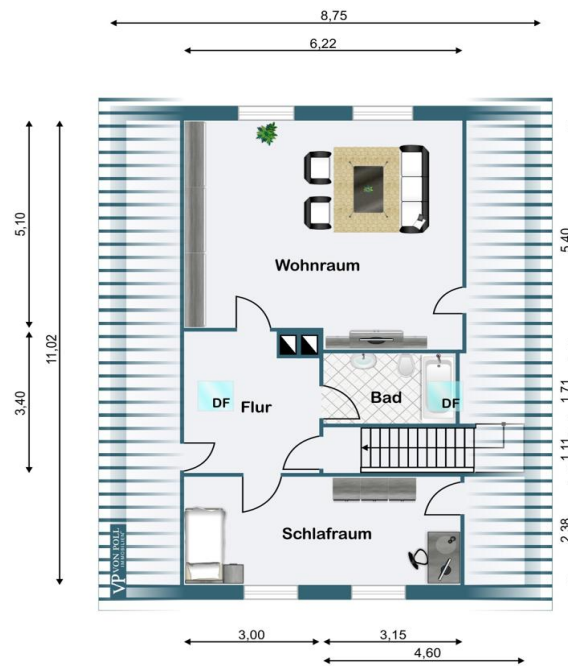
Dachgeschoss
