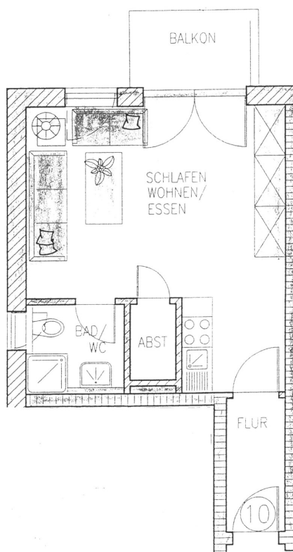
Obergeschoss 1
