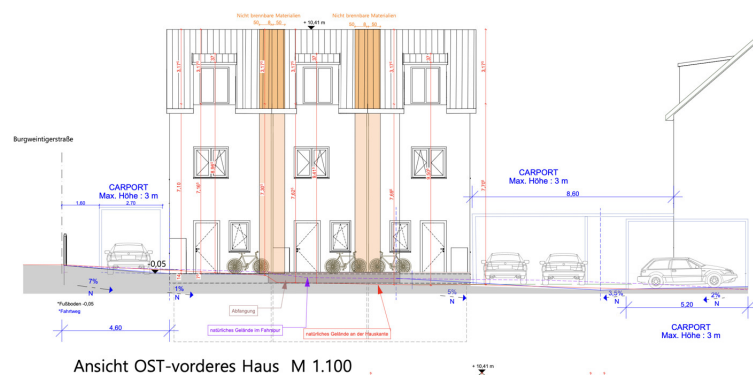
Ansicht OST-vorderes Haus M 1.100
