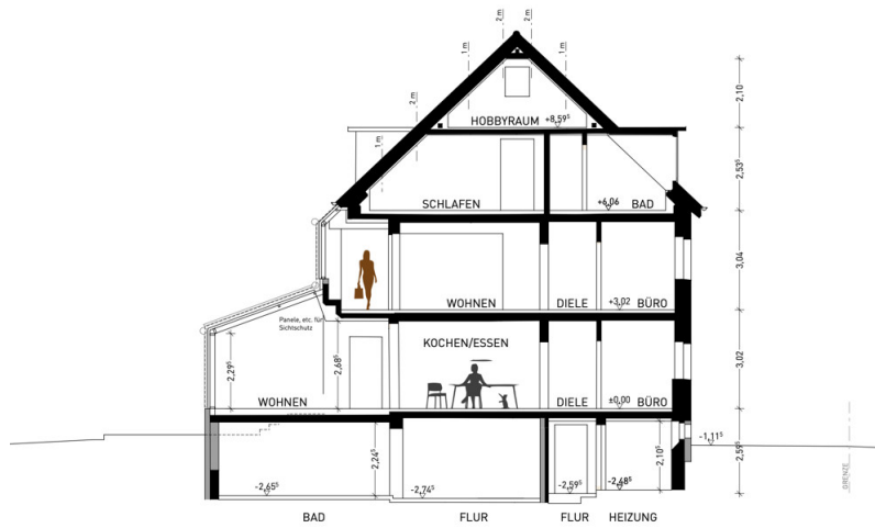
SCHNITT A-A
