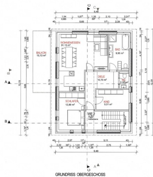
GRUNDRISS OBERGESCHOSS
