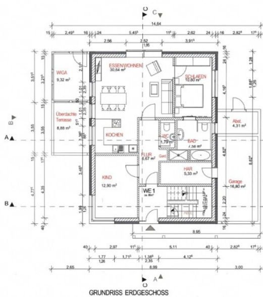
GRUNDRISS ERDGESCHOSS
