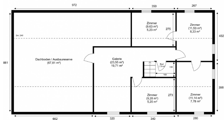
Dachgeschoss (Grundfläche)
