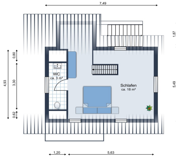
Dachgeschoss
