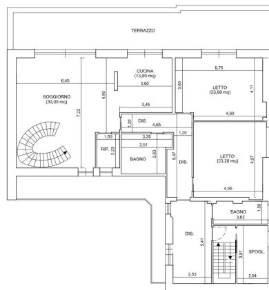
PIANTA PIANO QUARTO H = 3,45 m
