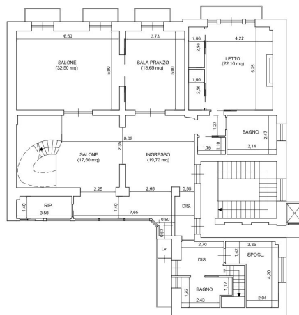
PIANTA PIANO TERZO H = 3,50 m
