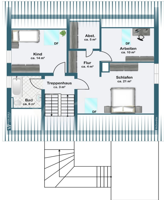
Dachgeschoss
