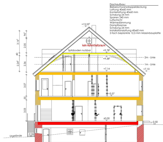
Schnitt A-A
