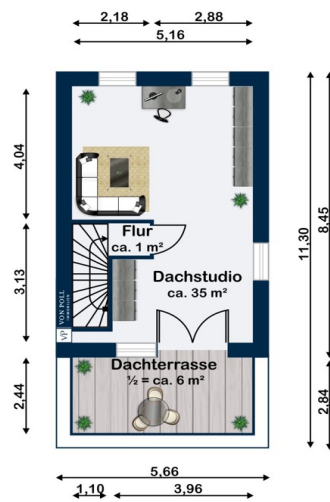
Dachgeschoss
