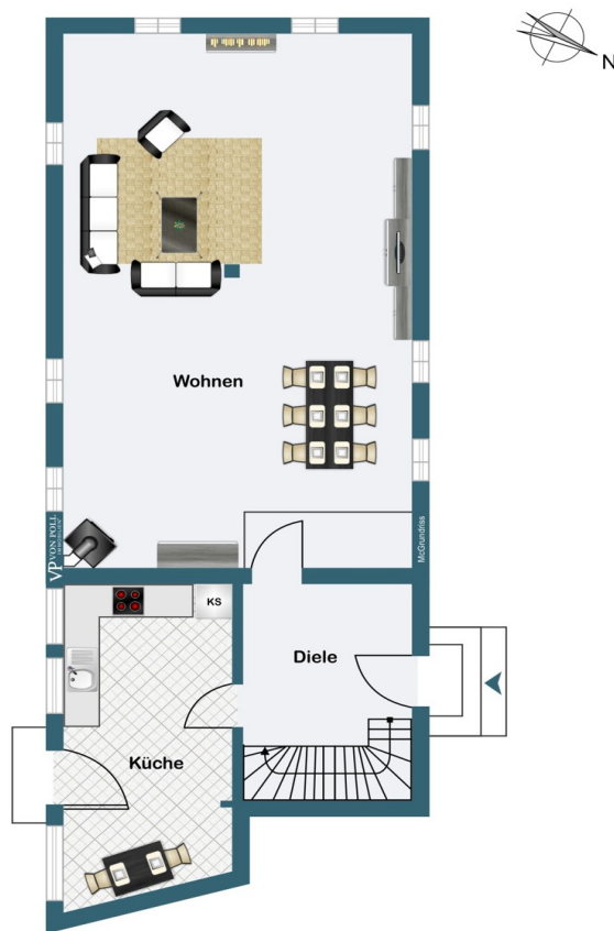
Erdgeschoss
