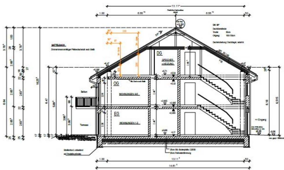
Schnitt B-B
