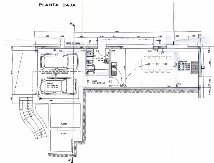
PLANTA SEMISOTANO
