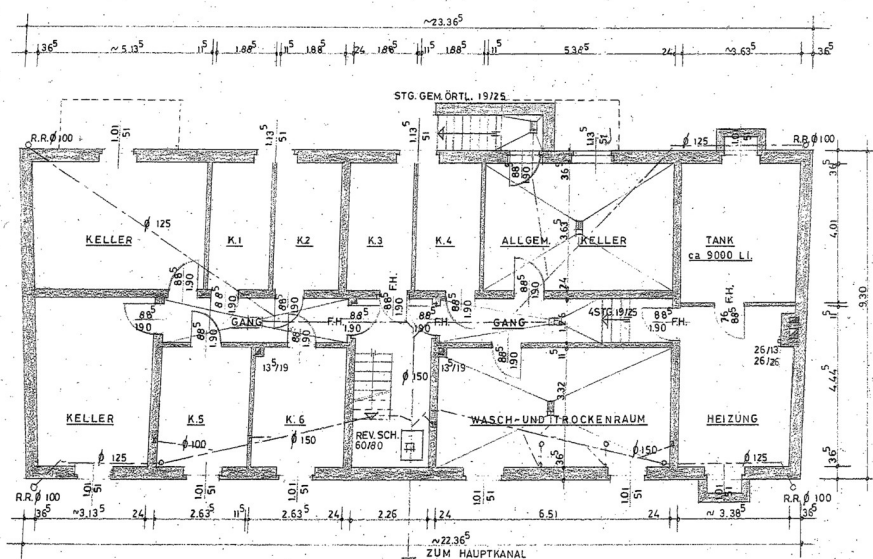
KELLERGESCHOSS M.1:100
