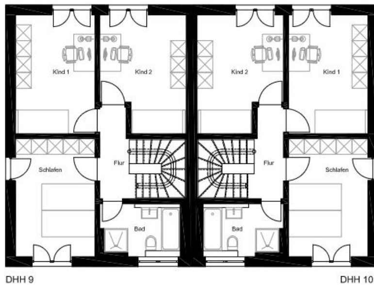
Grundriss OG
