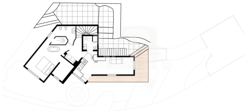
PRIMERA PLANTA
