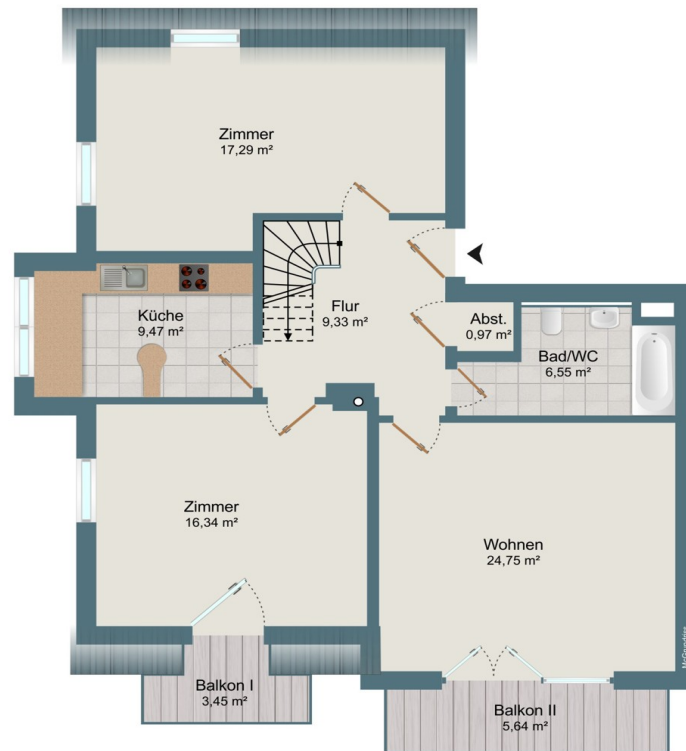
2. Obergeschoss
