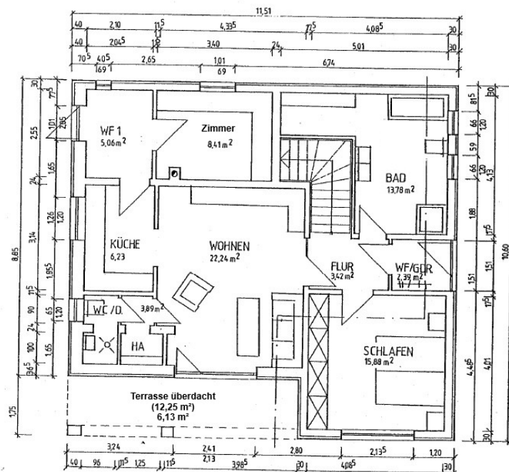
Erdgeschoss
