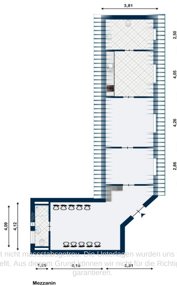
Mezzanin
