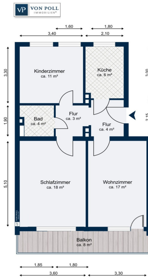
3. Obergeschoss
