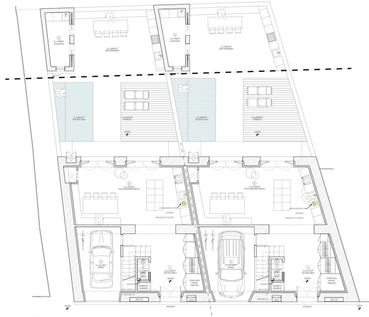
PLAN 000A (KARTELLIERUNG)
